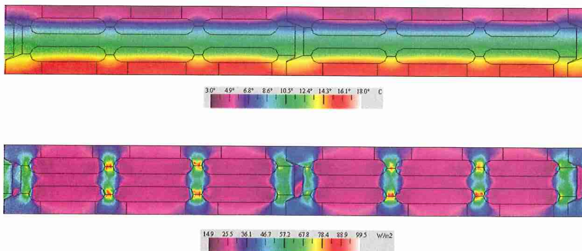
Fig. 5: Distribución de temperatura y flujo de calor en la fábrica de arliblock nº22, junto con las escalas correspondientes.
