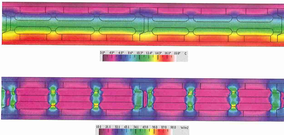
Fig. 6: Distribución de temperatura y flujo de calor en la fábrica de arliblock nº22 revestida, junto con las escalas correspondientes.
