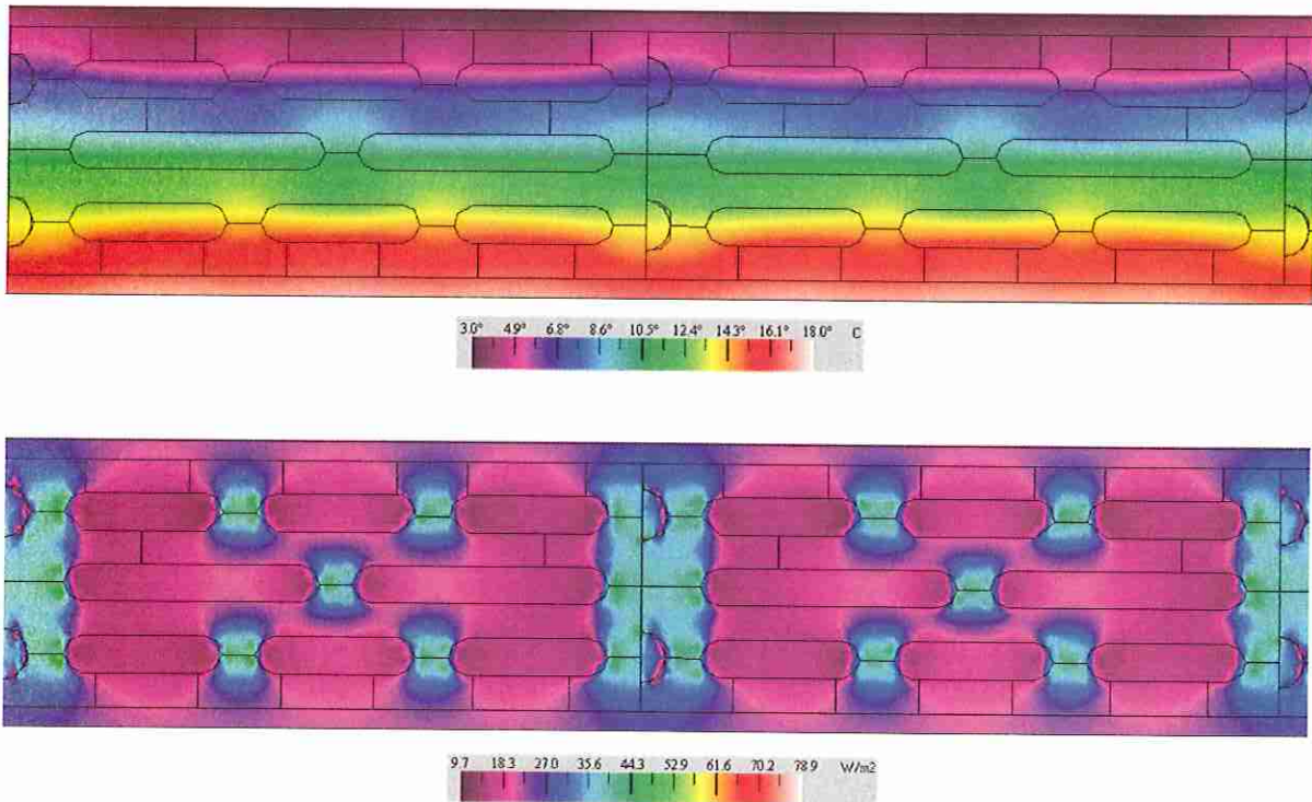
Fig. 4: Distribución de temperatura y flujo de calor en la fábrica de arliblock nº17 revestida, junto con las escalas correspondientes.
